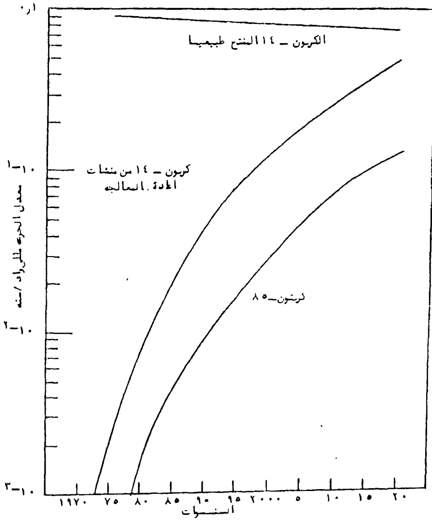
شكل (3): النشاط الاشعاعي للكربون 14 والكربون 13 المتراكم في الجو.
